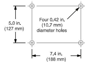
Szivattyútalp lukak
